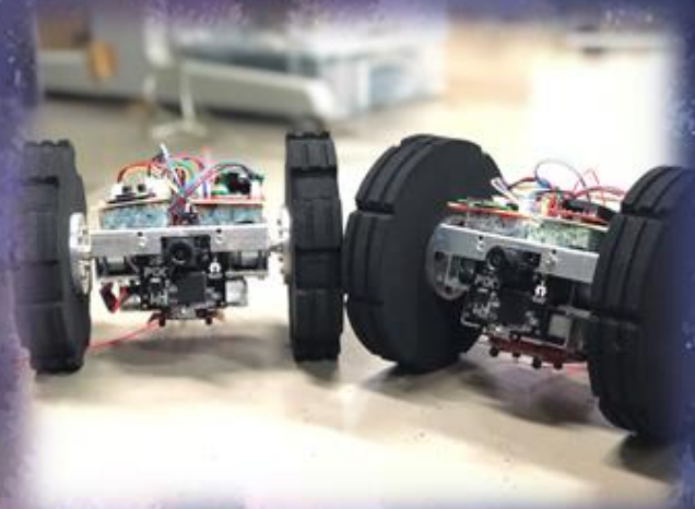
種子島ロケットコンテスト2018 製作したCan-Sat(カンサット)
